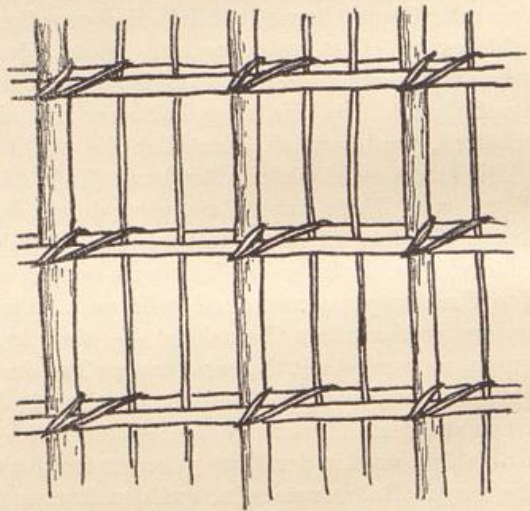
Fig. 22 Bindearbeit am Gerüst der Hauswand
