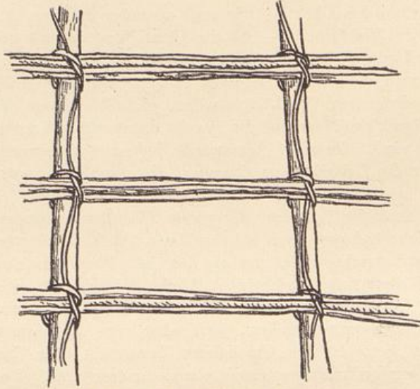
Fig. 21 Bindearbeit am Dachgerüst
