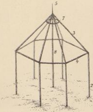
Kebu. Dachgerippe
