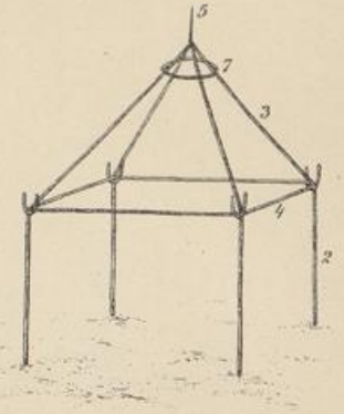
Akposso. Dachgerippe
