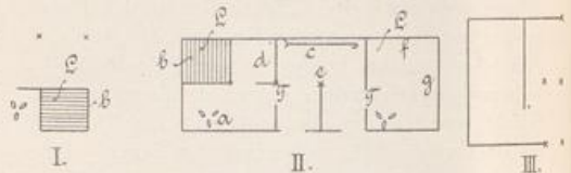
Fig. 8. Hütten aus dem Kral am N-Fuß des Hanang, Grundrisse, etwa 1:150.
