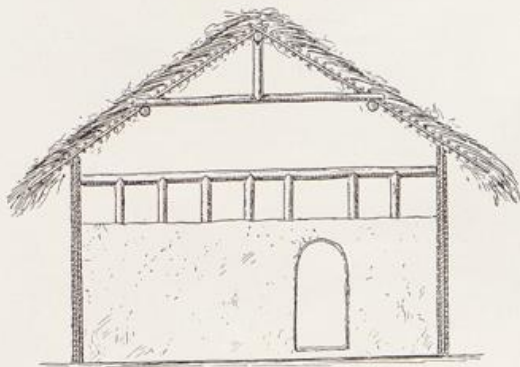
Abb. 2. Querwand im Innern eines Jaohauses in Tschingulungulu.
