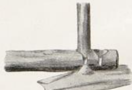
Abb. 7b. Einzelheit zu Fig. 7a
