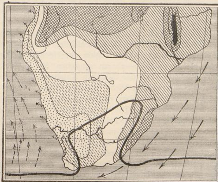
Karte 13. Jährliche Niederschlagsmenge.
