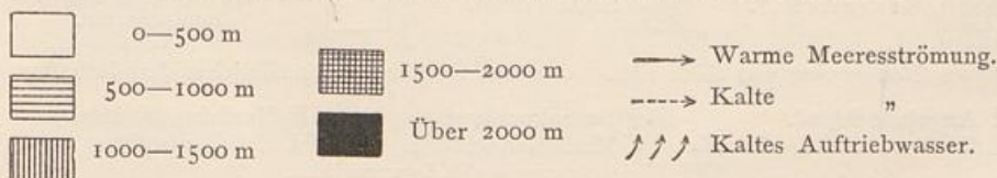
Karte 2. Orographische Skizze und Meeresströmungen.
