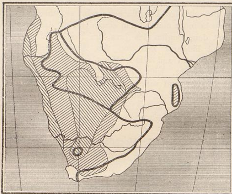
Karte 5. Wasserführung der Flüsse.
