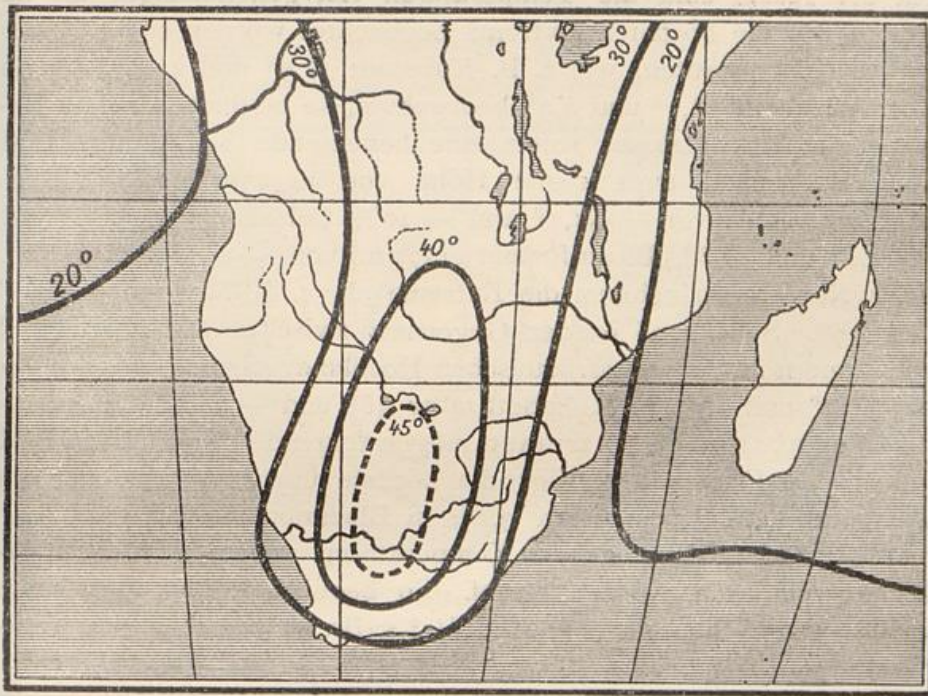
Karte 9. Mittlere absolute Jahresschwankungen der Temperatur (nach von Bebbber).
