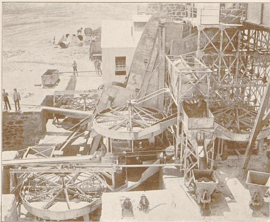
Die Maschinerie der De Beers Co. zum Sieben und Waschen der Diamanterde (Seite 279)
