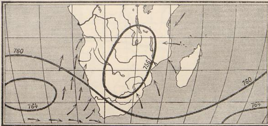
Karte 10. Januar-Isobaren (nach Hann).
