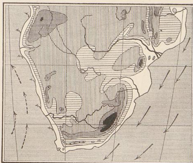
Karte 2. Orographische Skizze und Meeresströmungen.
