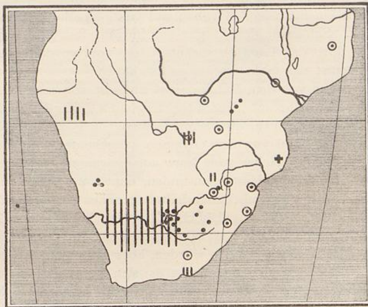
Karte 24. Mineralien (Nichtmetalle).
