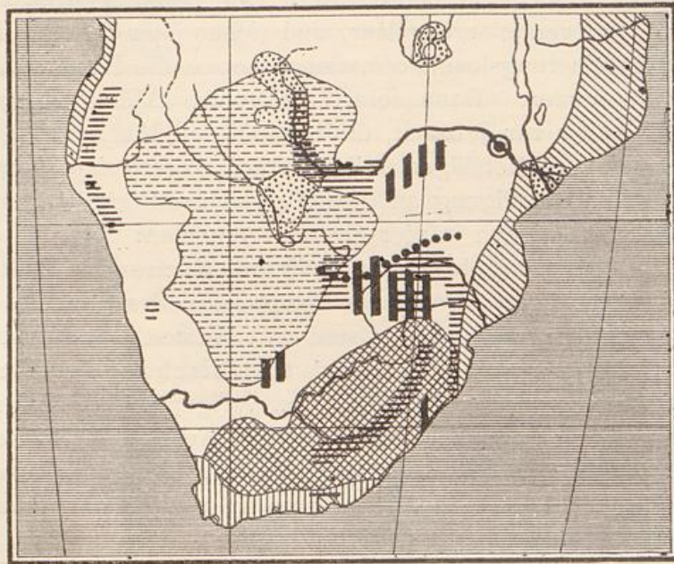
Karte 14. Geologische Skizze.
