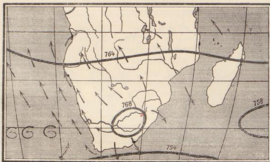
Karte 11. Juli-Isobaren (nach Hann).
