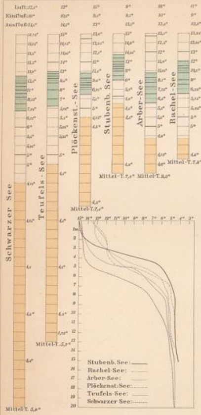
Temperaturen der Böhmerwald-Seen
