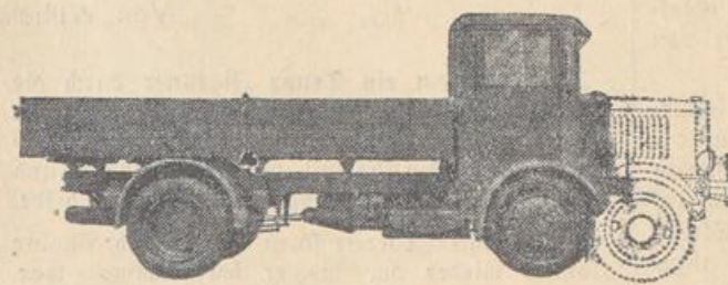
Der neuartige 3,5-t-Diesel-Lastwagen mit unter der Ladefläche liegendem Antriebsmotor. Zum Vergleich mit einem Lastwagen normaler Bauart ist der Motorvorbau und Kühler auf dem Bilde gestrichen.
