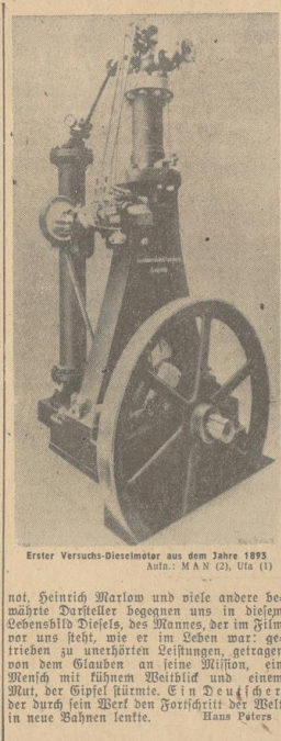
Erster Versuchs-Dieselmotor aus dem Jahre 1893
