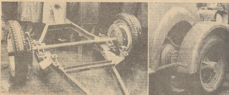
Links: Die Hilfsschleppprache, wie sie als Zusatzachse an den Personenwagen gebaut wird. Die Kraftübertragung erfolgt durch Zahnrad und Kette. Rechts: Die Hinterachse der Personenkraftwagen sind abgenommen und die Hilfsschleppprache ist eingebaut.
