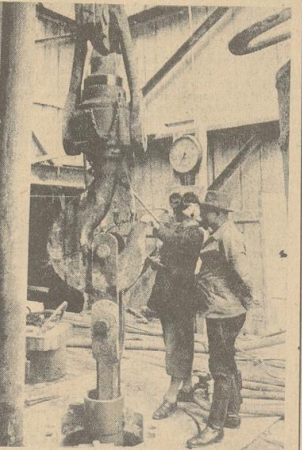
Der riesige Haken, an dem das Rohrgestänge hängt und mit dessen und des Mischensystems Hilfe immer neue Rohre nachgesetzt werden. Auf dem Bild unten ist die durchstanzte Tellerschibe sichtbar, die das ganze Bohrgestänge in Rotation versetzt.
