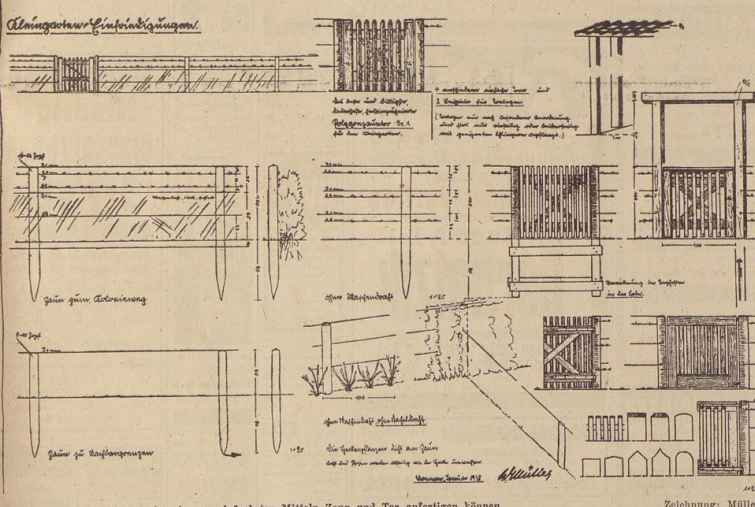
Diese Skizzen zeigen, wie wir aus einfachen Mitteln Zaun und Tor anfertigen können.
