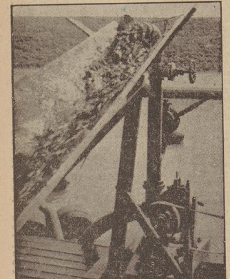
In dickem Strahl wirft die Pumpenöffnung Schlamm und Wasser heraus. Aufnahmen: Sant (2).
