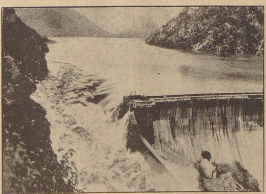
Riesiger Staudamm in Australien in Gefahr. Ein breiter Riß zeigte sich in dem riesigen Burrinjuck Staudamm in der australischen Provinz Neu-Süd-Wales. Alle zur Verfügung stehenden Arbeitskräfte arbeiten zur Zeit daran, den Staudamm wieder abzudichten. Unser Bild zeigt, wie das Wasser durch die breite Bruchstelle strömt. (Presse-Hoffmann).
