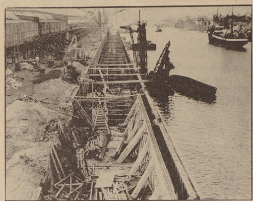
Unser Bild, das einen Blick über die gegenwärtige Baustelle gewährt, veranschaulicht deutlich die Art der Verbreiterung des Piers. Aufn.: Bors (2)
