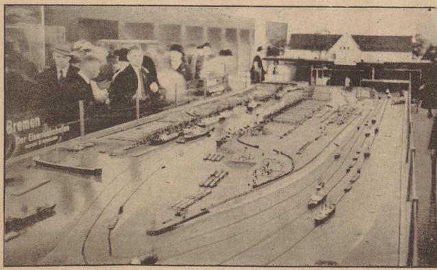
Ueber Größe und Bedeutung der bremischen Hafenanlagen gibt den zahllosen Besuchern aus allen Gauen Deutschlands das bewegliche Modell einer Teilanlage des größten deutschen Eisenbahnhafens Auskunft. Unser Bild zeigt die Hafenbecken des Freihafens I und II sowie das Wendebassin. Im Vordergrund (links) ein Schiff im Dock der A.G. „Weser“ (Aufn.: Schmidt (7))
