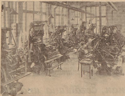
In langen Reihen stehen die Setzmaschinen. Hier wird das geschriebene Wort in Blei gegossen
