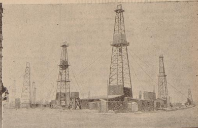
In dem bekannten Erdölgebiet Kienhagen in Hannover hielt man auf große Erdölfontänen. Unter einem Druck von 6 Atmosphären entströmen einer Düse von 25 mm Durchmesser täglich 200 Tonnen Erdöl. Es ist dies ein Rekord, der in der deutschen Erdölproduktion noch nicht erreicht worden ist.
